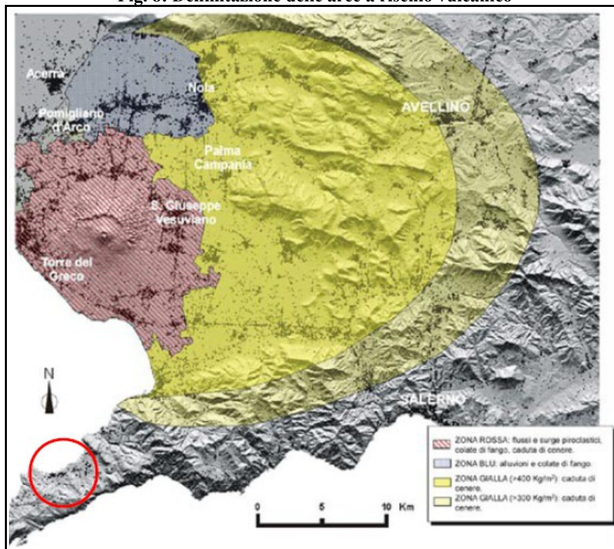
Fig. 9: Delimitazione delle aree a rischio vulcanico con indicazione del settore in cui è inserito il territorio comunale di Meta .
